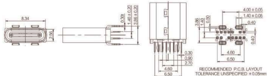
TYPE-C 14P-F 立式贴片SMT缩口 H=8.20mm
