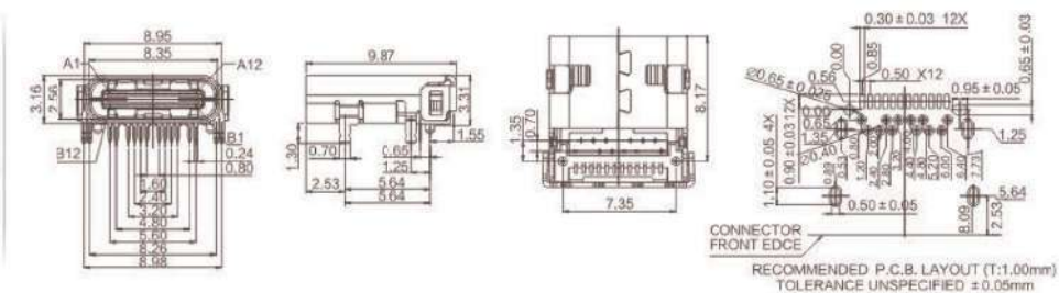
TYPE-C 24P-F 板上四脚插板DIP+SMT 无弹片 L=8.65 / 10.0mm
