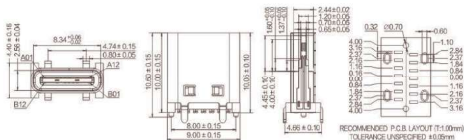
TYPE-C 14P-F 双层立式直插DIP H=11.0mm
