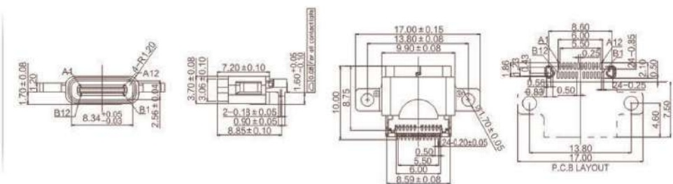
防水TYPE-C 24P-F 沉板1.6锁板式双SMT L=9.60mm
