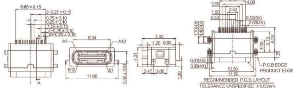
防水TYPE-C 24P-F 沉板1.0前贴后插DIP+SMT一体式外壳 L=9.0mm
