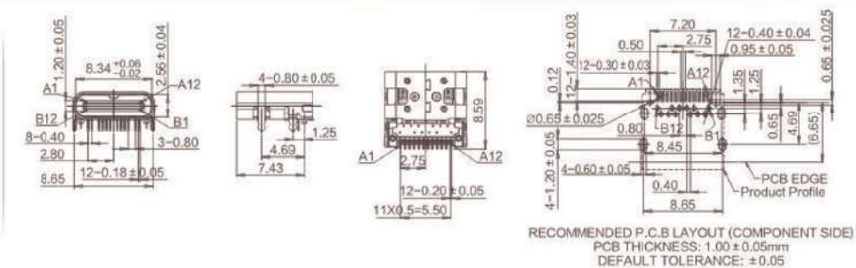
TYPE-C 24P-F 板上四腳插板DIP+SMT帶彈片 L=9.87mm
