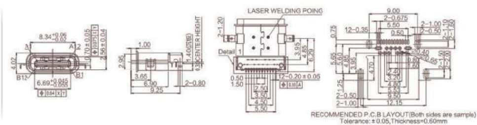
防水TYPE-C 24P-F 沉板1.6锁板式双SMT L=9.60mm
