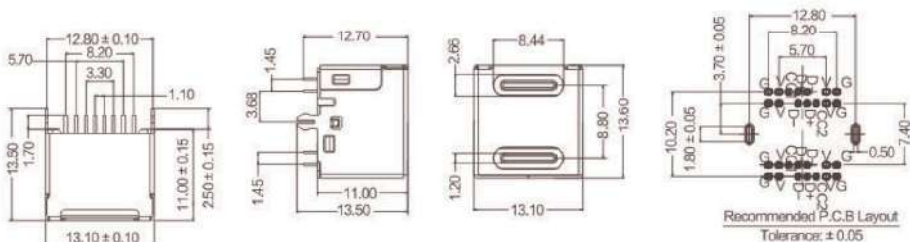
TYPE-C 14P-F 双层立式直插DIP H=11.0mm
